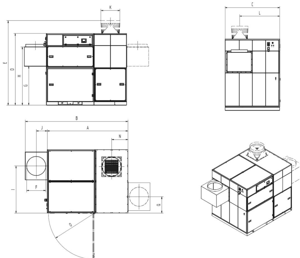
Rys. 56: Karta wymiarów 998701370 (998800414, 998800463)
