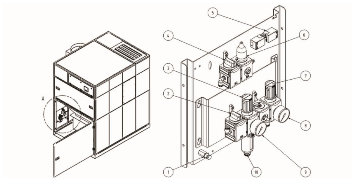
Rys. 10: Stacja sprężonego powietrza
