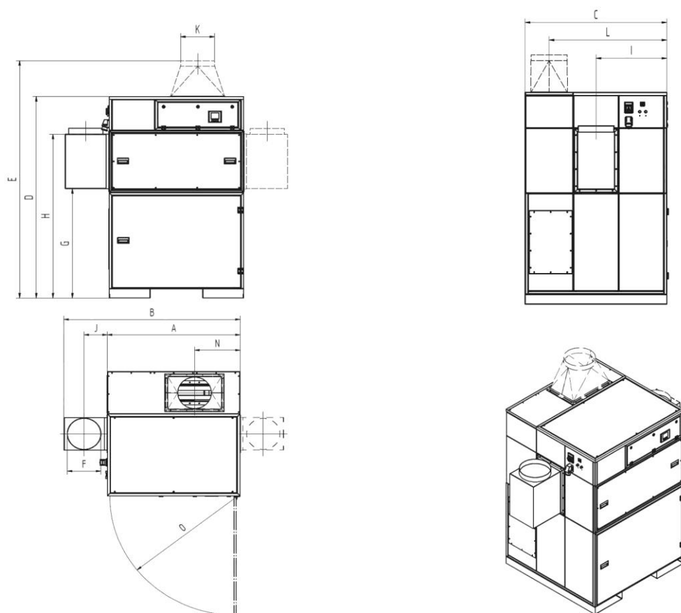
Rys. 54: Karta wymiarów 998701372 (998800407, 998800461)
